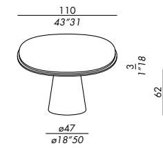
tavolo - table LOUNGE
