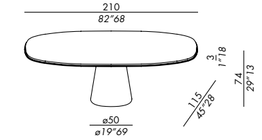
tavolo - table TP-210115
