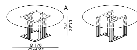
tavolo - table 170R-TP
