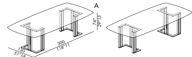
tavolo - table 130300-TP
